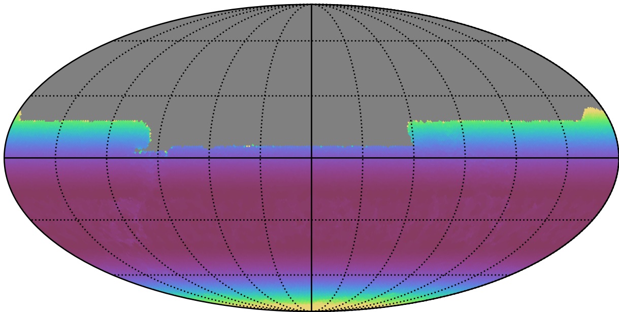
no_long_daily_v3.4_10yrs All sky y band: Min airmass
