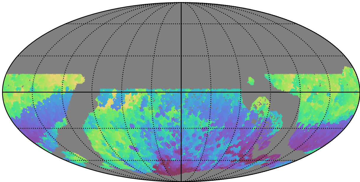
no_long_daily_v3.4_10yrs WFD z band: Min HA
