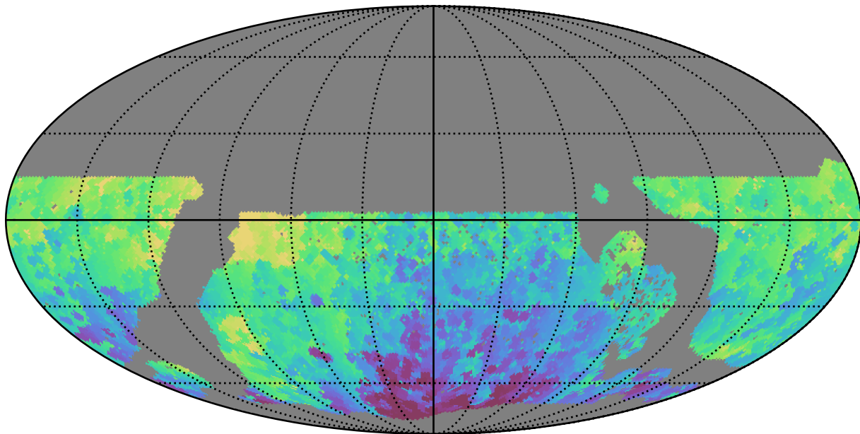
no_long_daily_v3.4_10yrs WFD y band: Min HA
