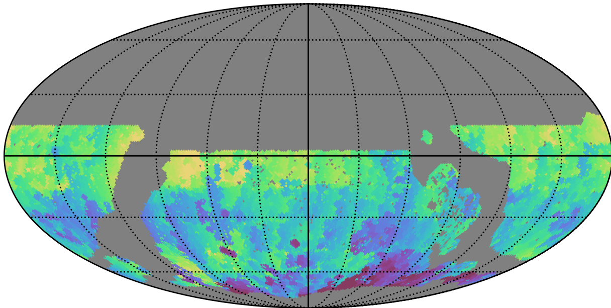
no_long_daily_v3.4_10yrs WFD u band: Min HA
