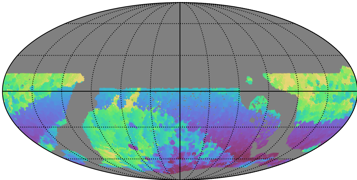
no_long_daily_v3.4_10yrs WFD r band: Min HA
