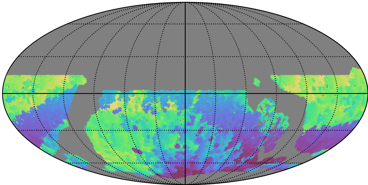
no_long_daily_v3.4_10yrs WFD i band: Min HA
