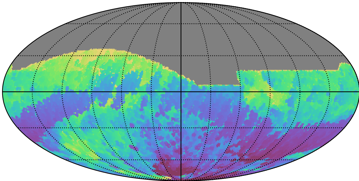
no_long_daily_v3.4_10yrs All sky z band: Min HA
