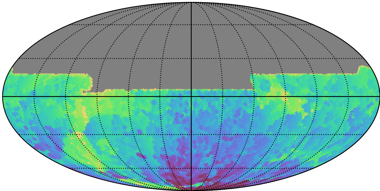
no_long_daily_v3.4_10yrs All sky y band: Min HA
