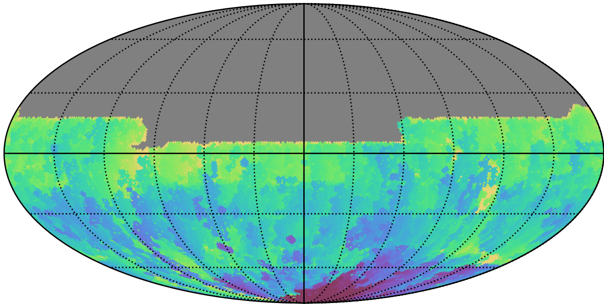
no_long_daily_v3.4_10yrs All sky u band: Min HA
