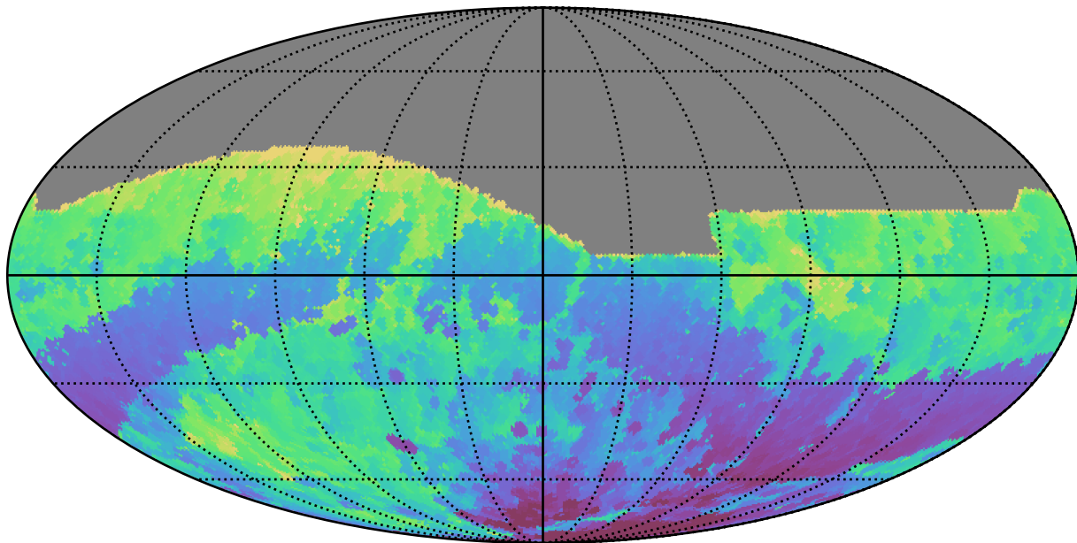
no_long_daily_v3.4_10yrs All sky i band: Min HA
