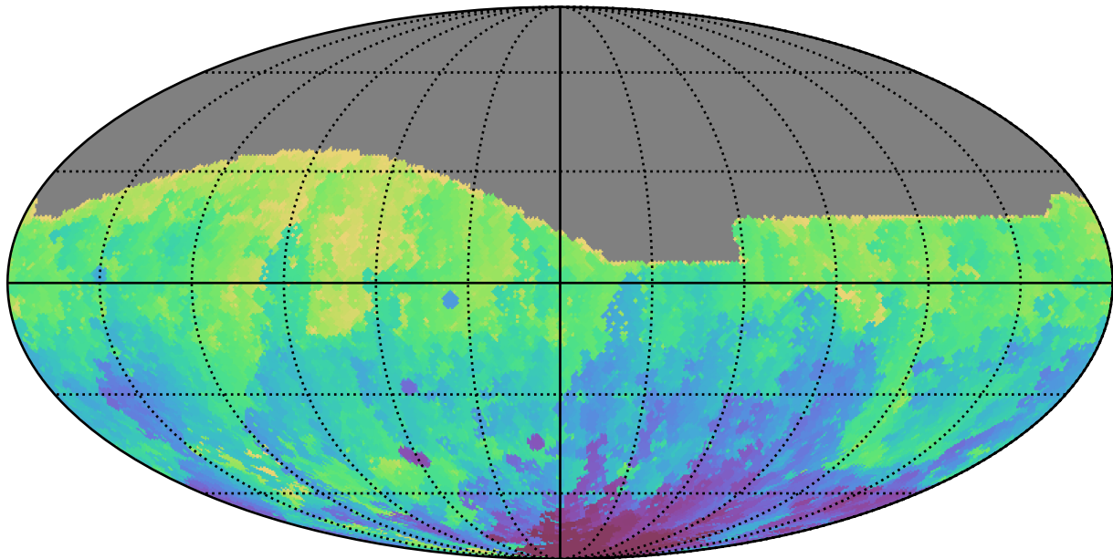
no_long_daily_v3.4_10yrs All sky g band: Min HA
