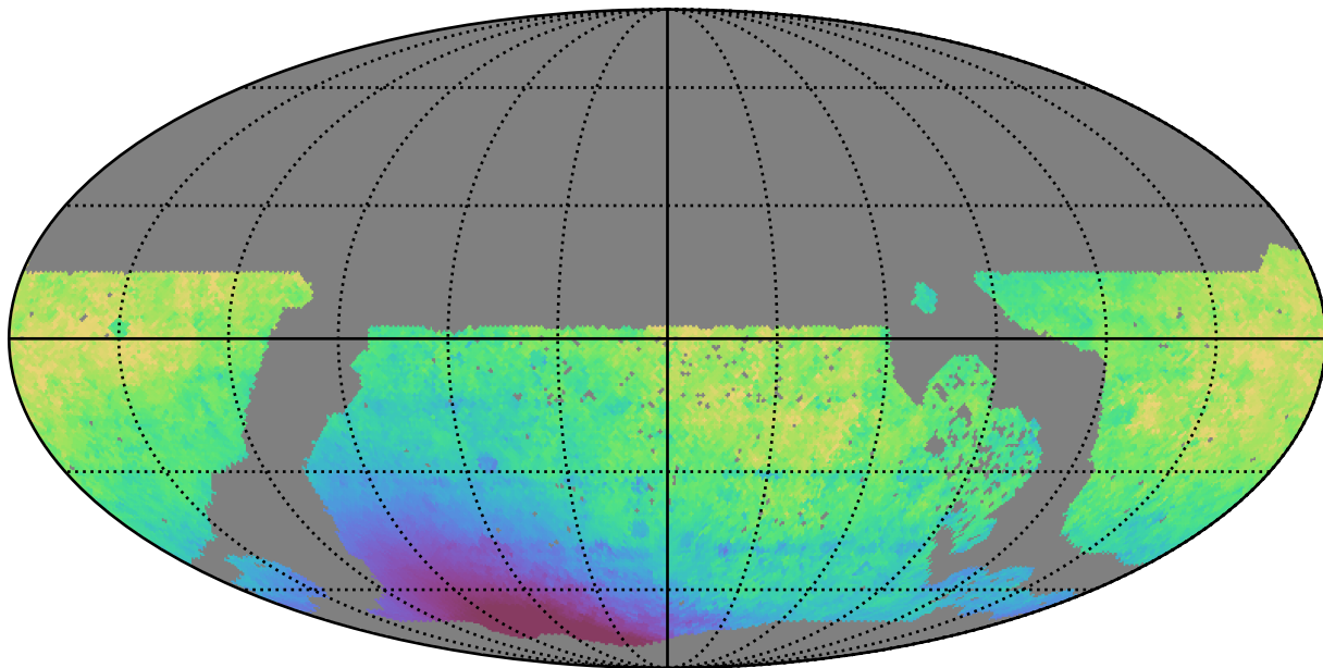
no_long_daily_v3.4_10yrs WFD z band: Median solarElong
