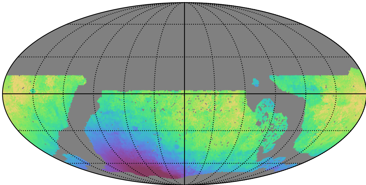
no_long_daily_v3.4_10yrs WFD y band: Median solarElong
