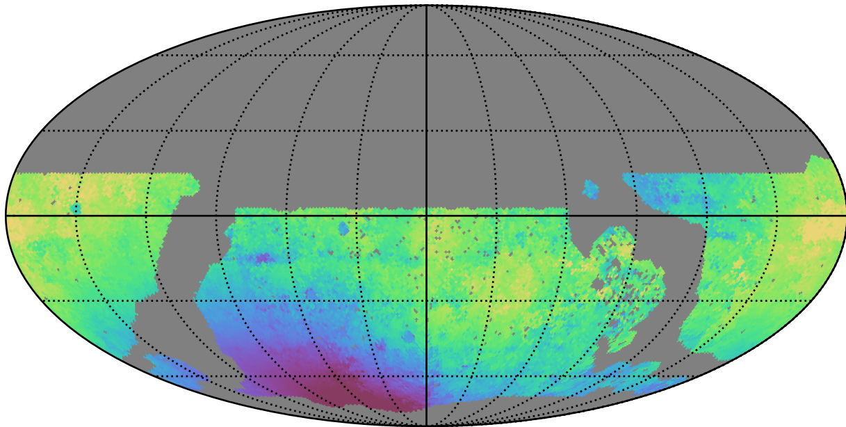
no_long_daily_v3.4_10yrs WFD u band: Median solarElong
