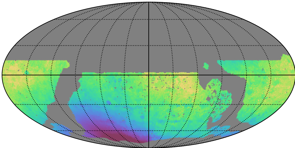
no_long_daily_v3.4_10yrs WFD i band: Median solarElong
