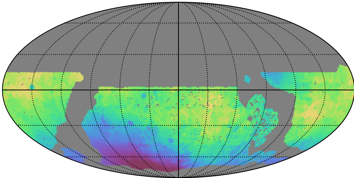
no_long_daily_v3.4_10yrs WFD g band: Median solarElong
