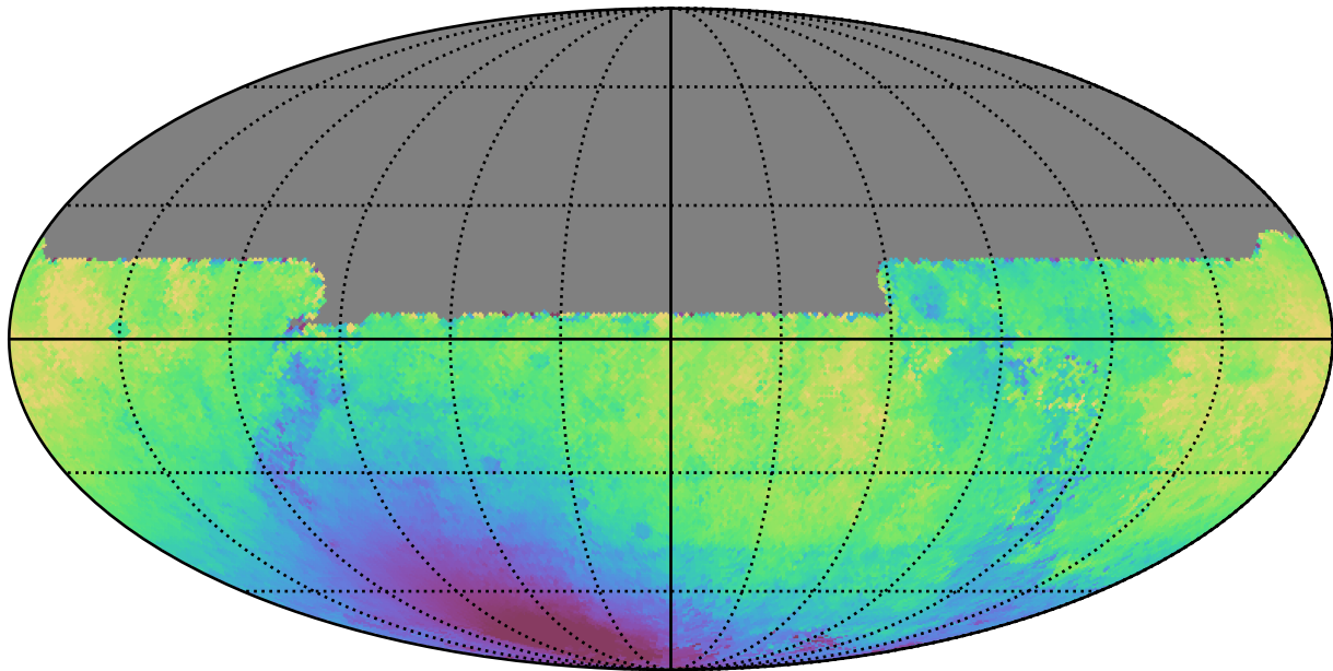
no_long_daily_v3.4_10yrs All sky y band: Median solarElong
