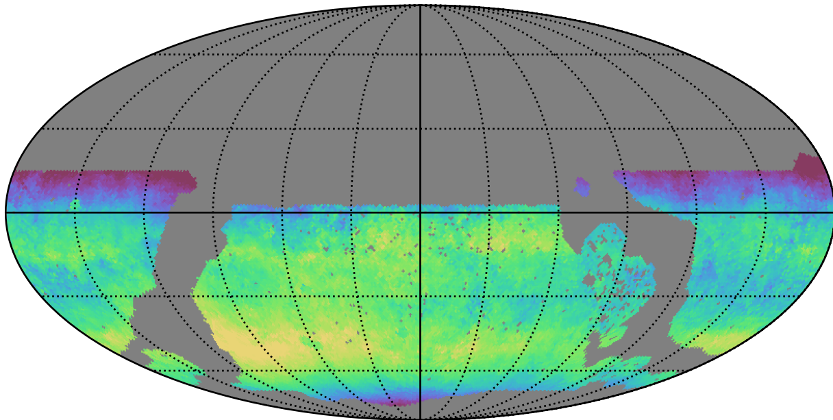
no_long_daily_v3.4_10yrs WFD y band: Median skyBrightness
