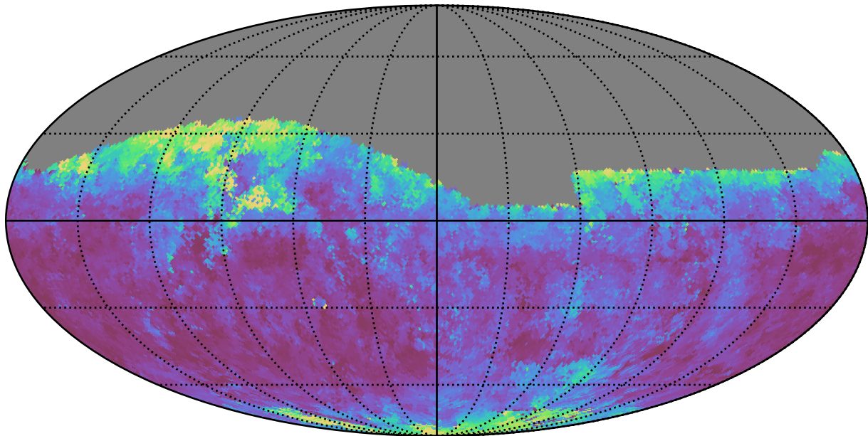
no_long_daily_v3.4_10yrs Yr 1 i band: Median seeingGeom
