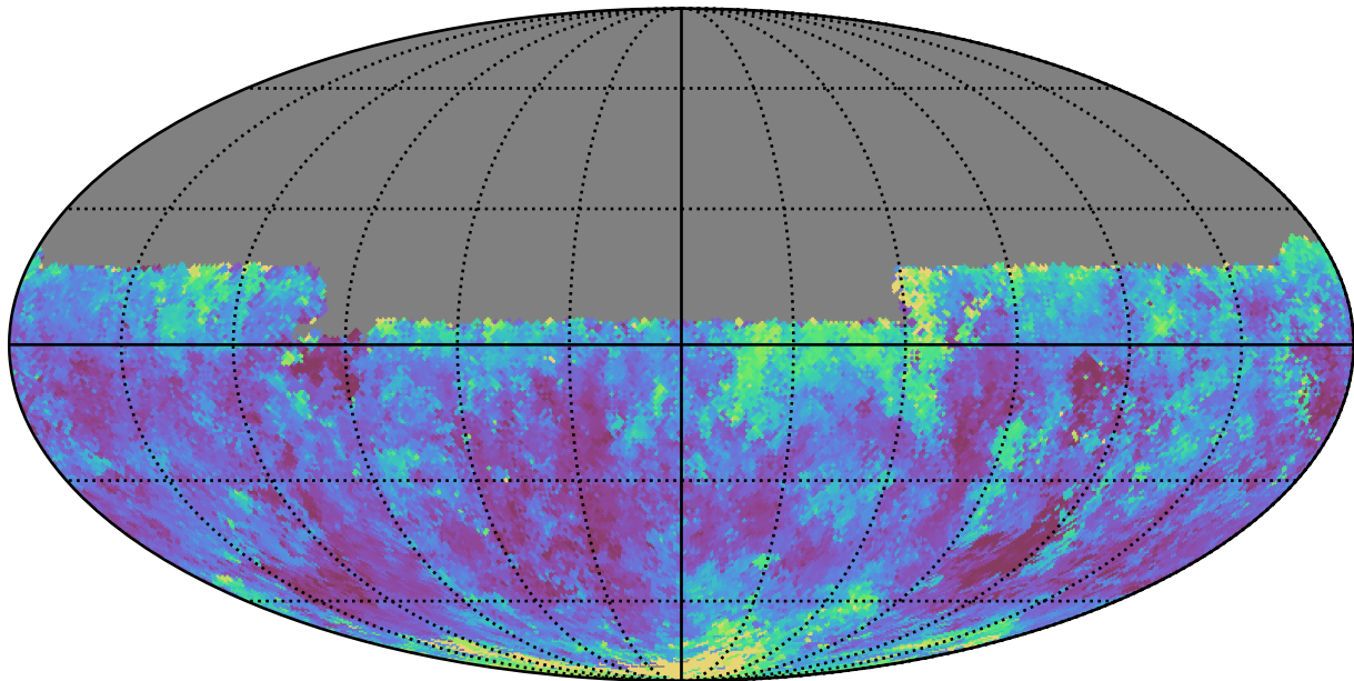
no_long_daily_v3.4_10yrs Yr 1 y band: Median seeingEff
