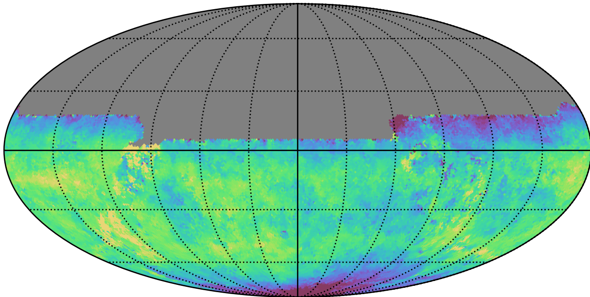
no_long_daily_v3.4_10yrs All sky u band: Median saturation_mag
