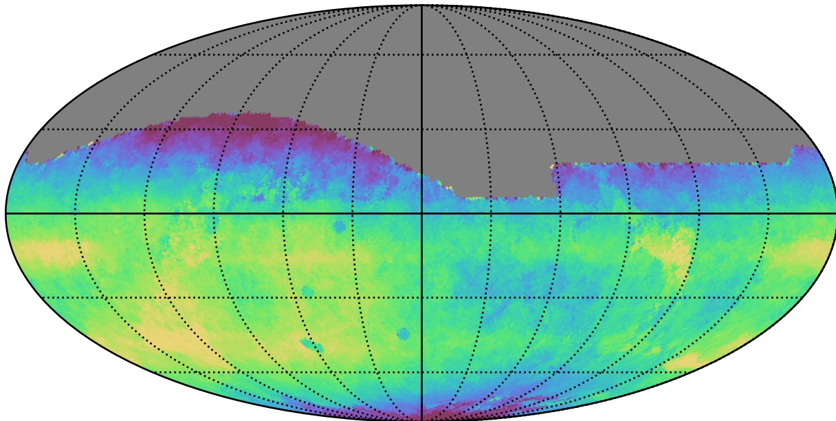
no_long_daily_v3.4_10yrs All sky r band: Median saturation_mag
