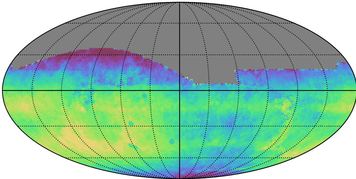
no_long_daily_v3.4_10yrs All sky i band: Median saturation_mag
