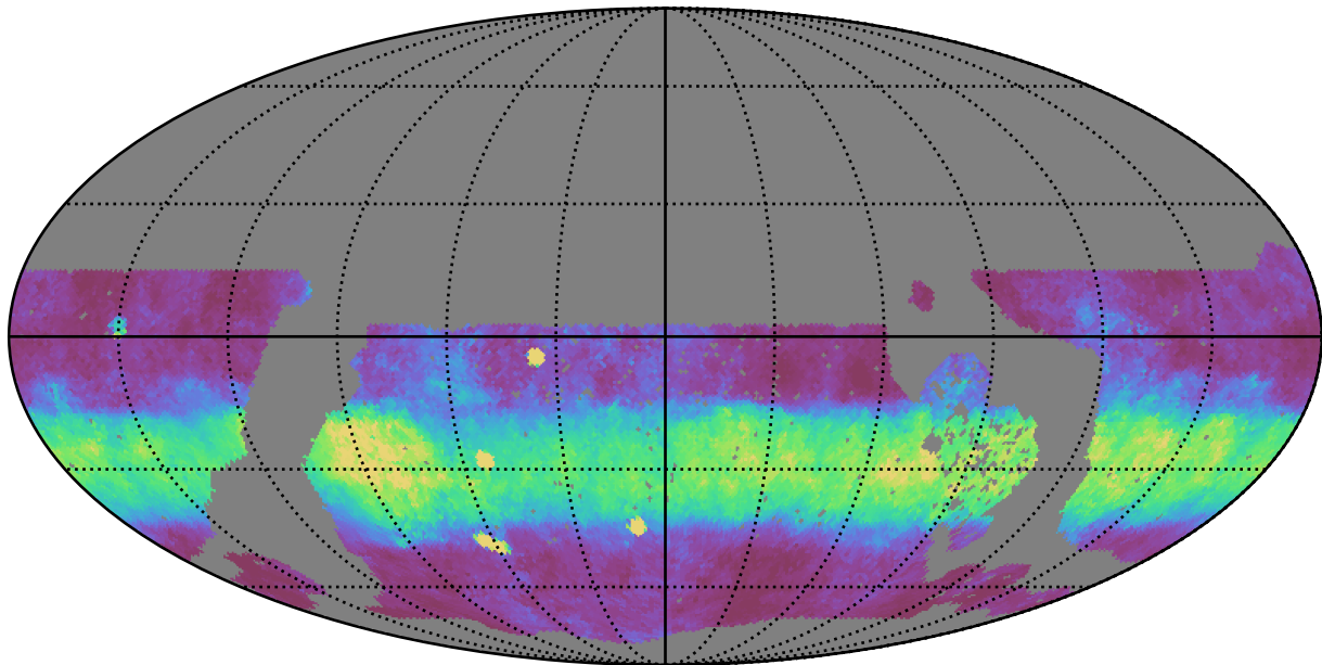
no_long_daily_v3.4_10yrs WFD y band: Median normairmass
