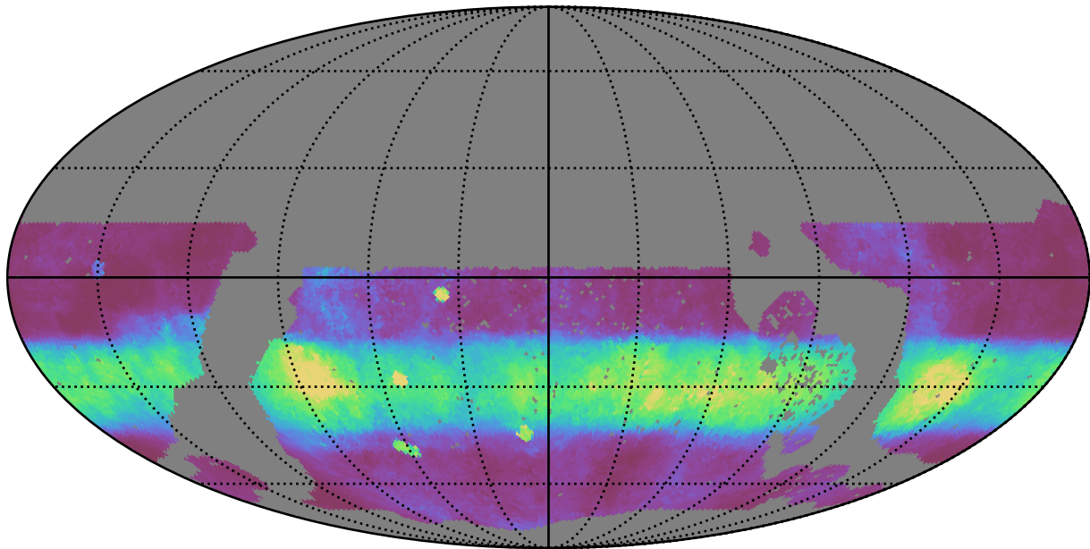
no_long_daily_v3.4_10yrs WFD r band: Median normairmass
