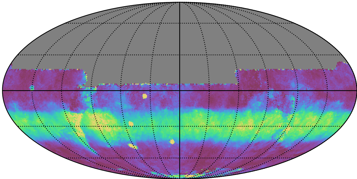
no_long_daily_v3.4_10yrs All sky y band: Median normairmass
