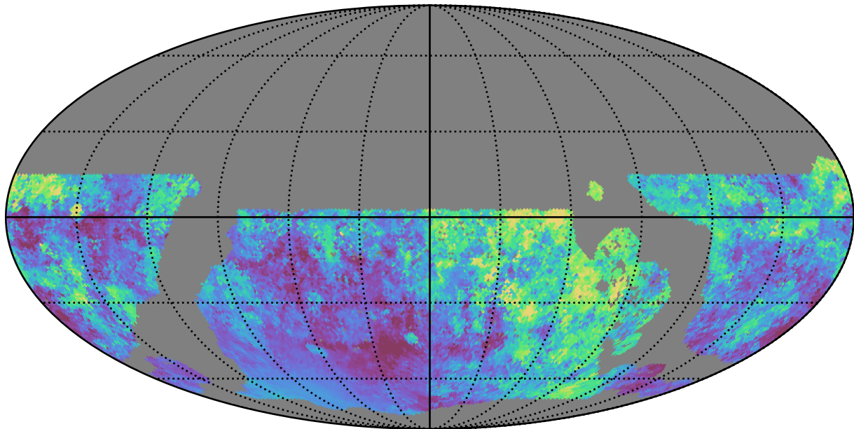
no_long_daily_v3.4_10yrs WFD i band: Median moonDistance
