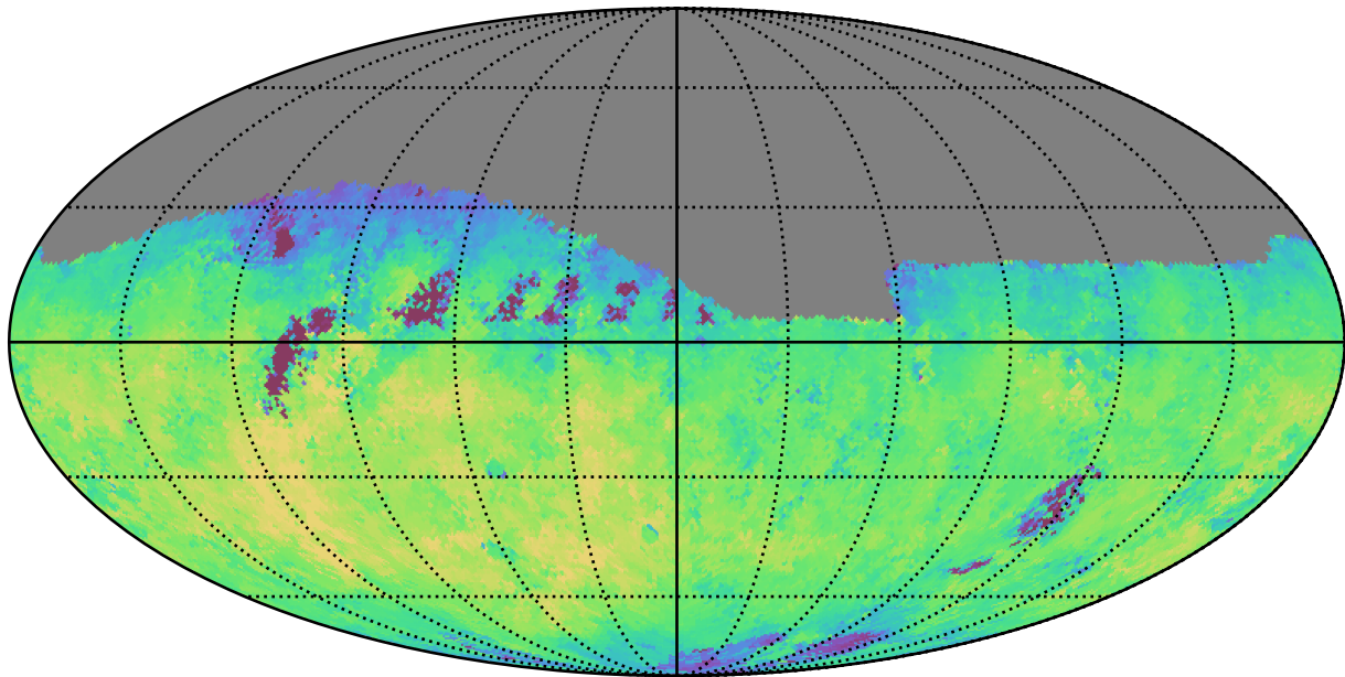
no_long_daily_v3.4_10yrs Yr 1 r band: Median fiveSigmaDepth
