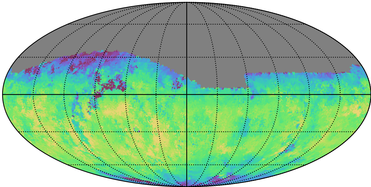
no_long_daily_v3.4_10yrs Yr 1 i band: Median fiveSigmaDepth
