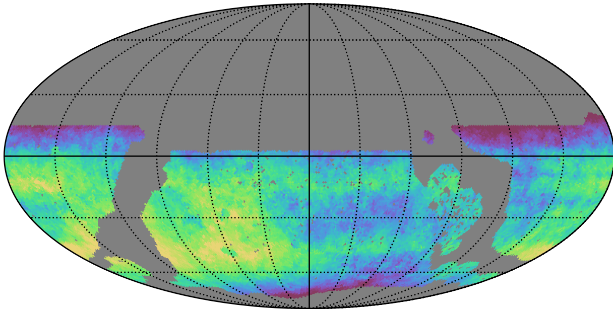
no_long_daily_v3.4_10yrs WFD z band: Median fiveSigmaDepth
