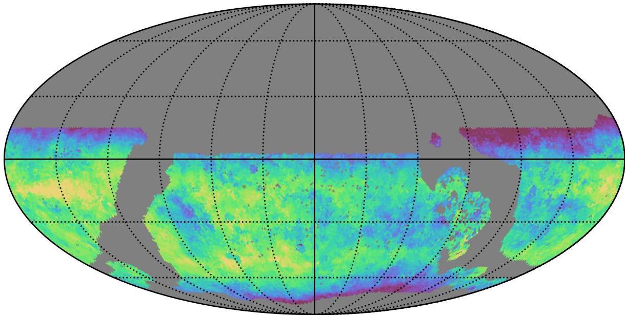
no_long_daily_v3.4_10yrs WFD u band: Median fiveSigmaDepth
