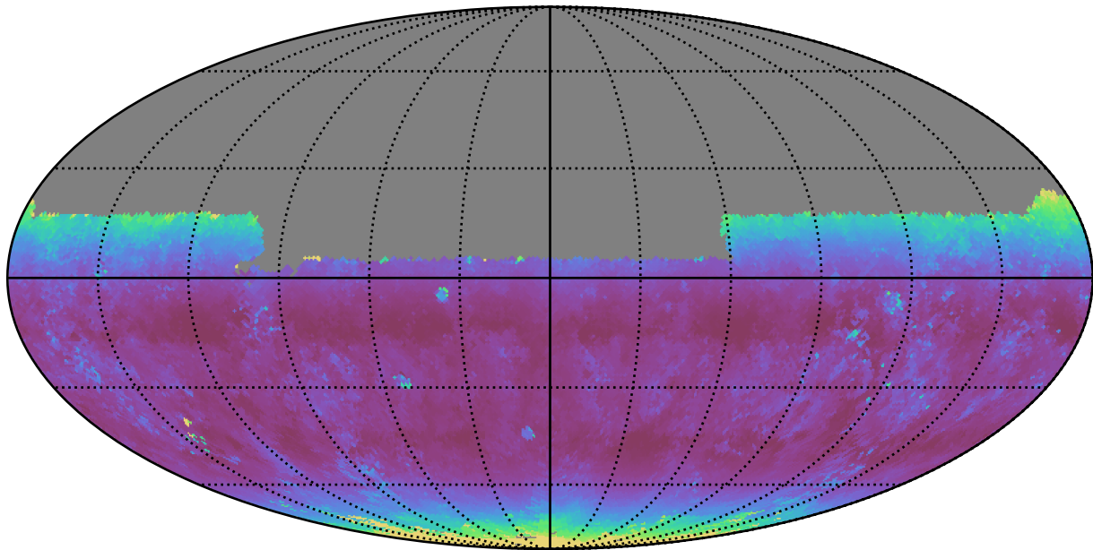
no_long_daily_v3.4_10yrs Yr 1 y band: Median airmass
