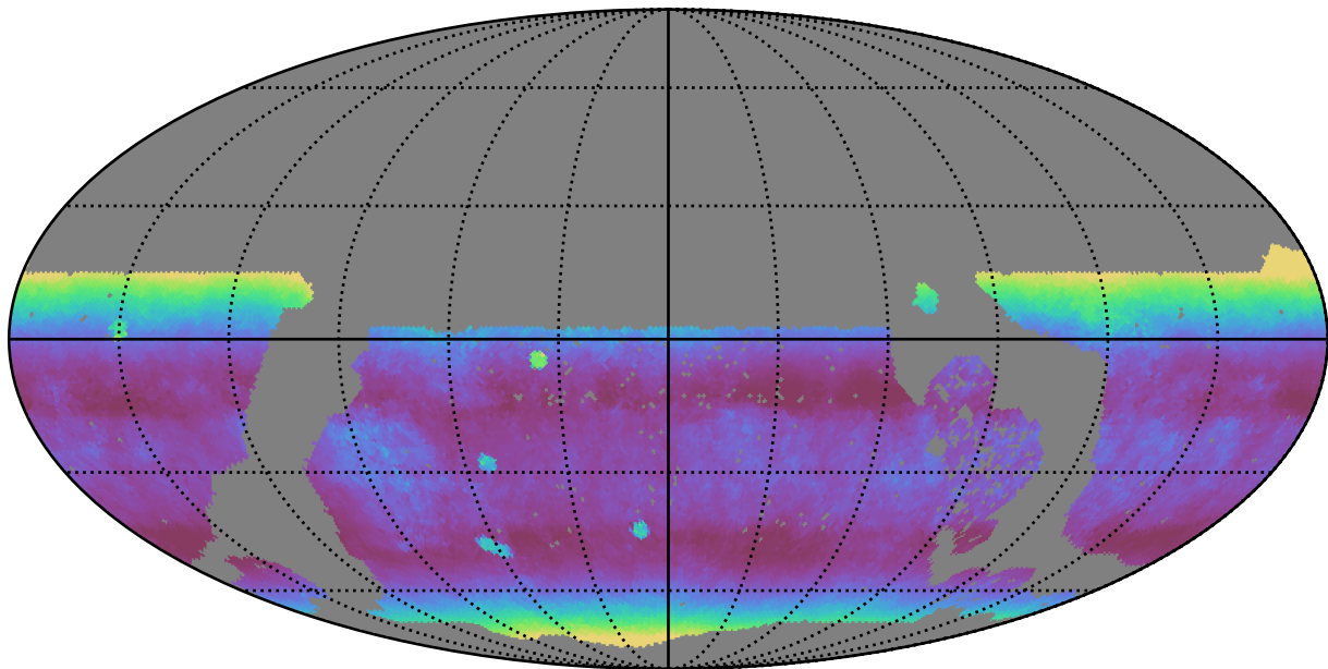
no_long_daily_v3.4_10yrs WFD y band: Median airmass
