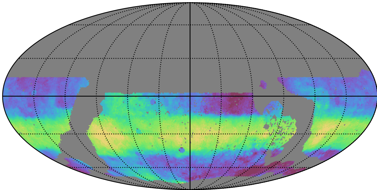
no_long_daily_v3.4_10yrs WFD z band: Median HA
