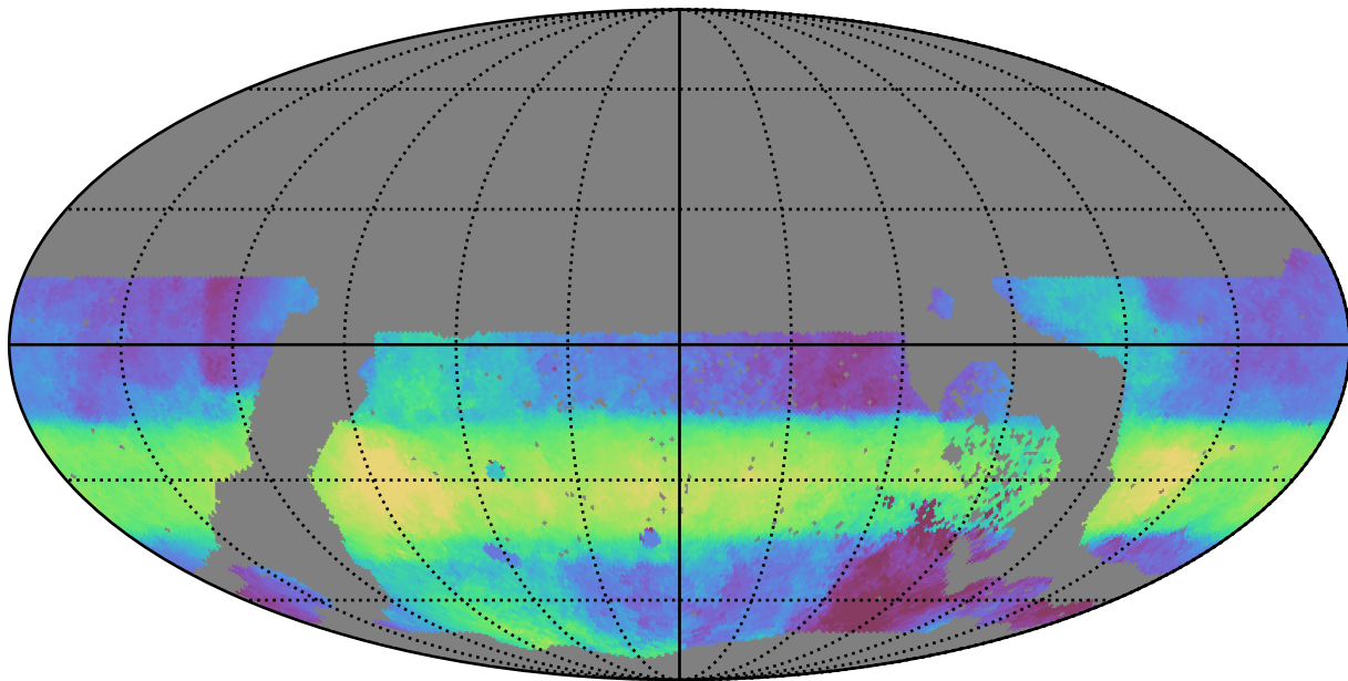
no_long_daily_v3.4_10yrs WFD r band: Median HA
