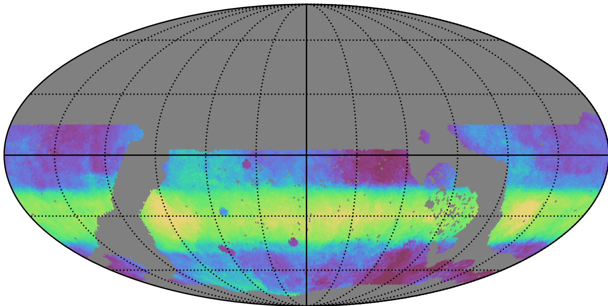
no_long_daily_v3.4_10yrs WFD i band: Median HA
