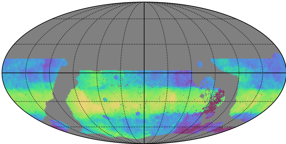
no_long_daily_v3.4_10yrs WFD g band: Median HA
