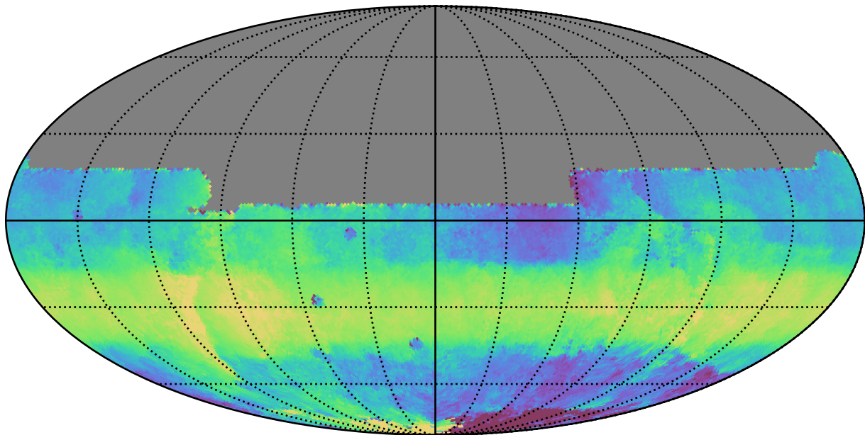
no_long_daily_v3.4_10yrs All sky y band: Median HA
