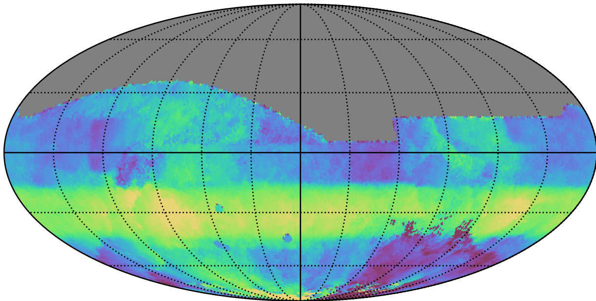
no_long_daily_v3.4_10yrs All sky r band: Median HA
