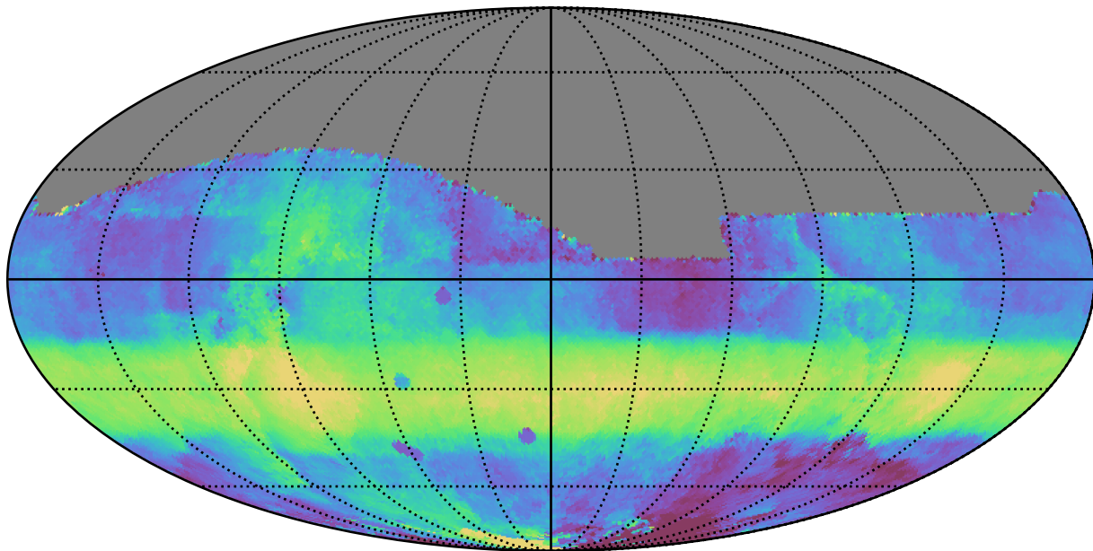
no_long_daily_v3.4_10yrs All sky i band: Median HA
