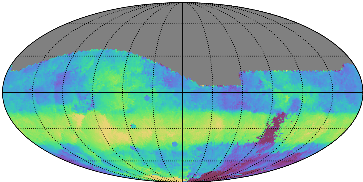
no_long_daily_v3.4_10yrs All sky g band: Median HA
