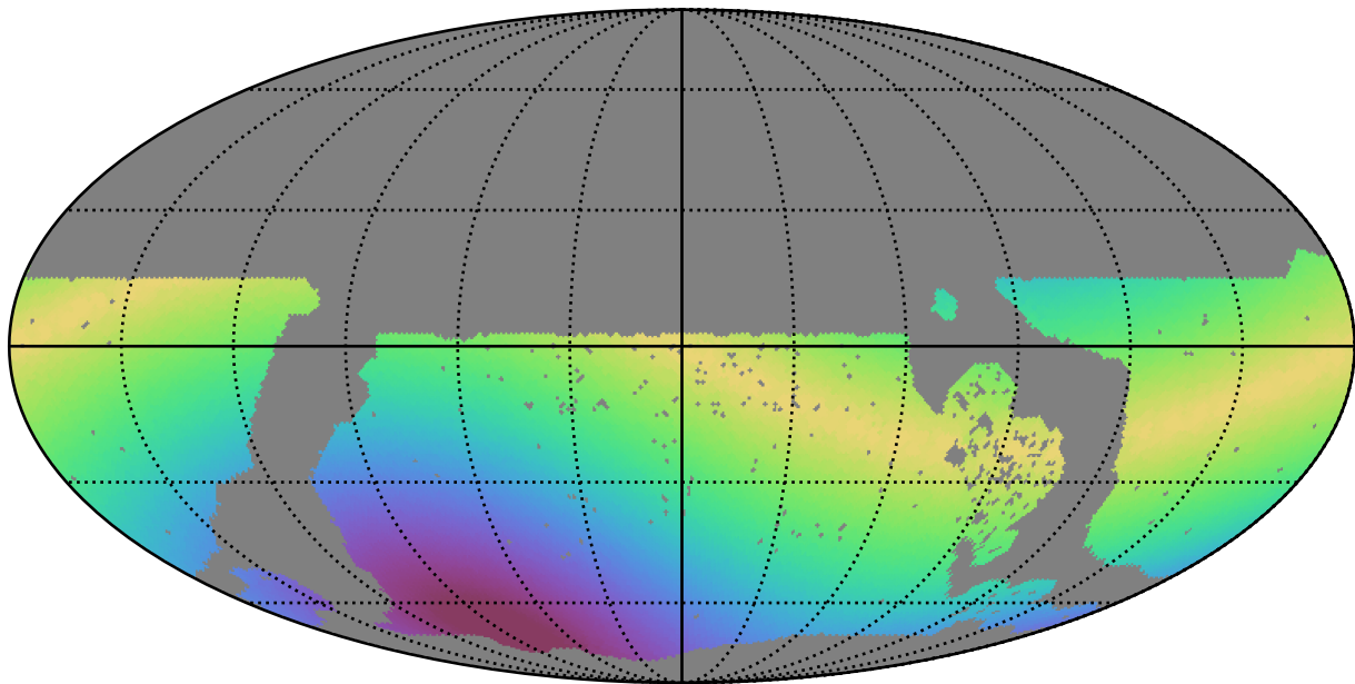
no_long_daily_v3.4_10yrs WFD y band: Max solarElong
