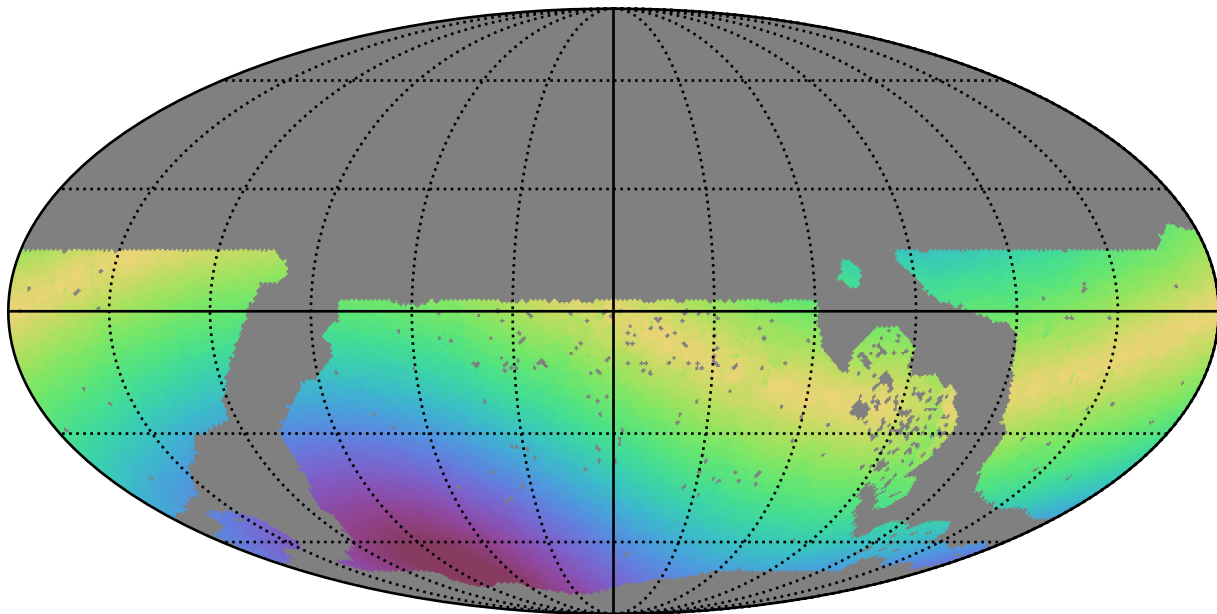
no_long_daily_v3.4_10yrs WFD u band: Max solarElong
