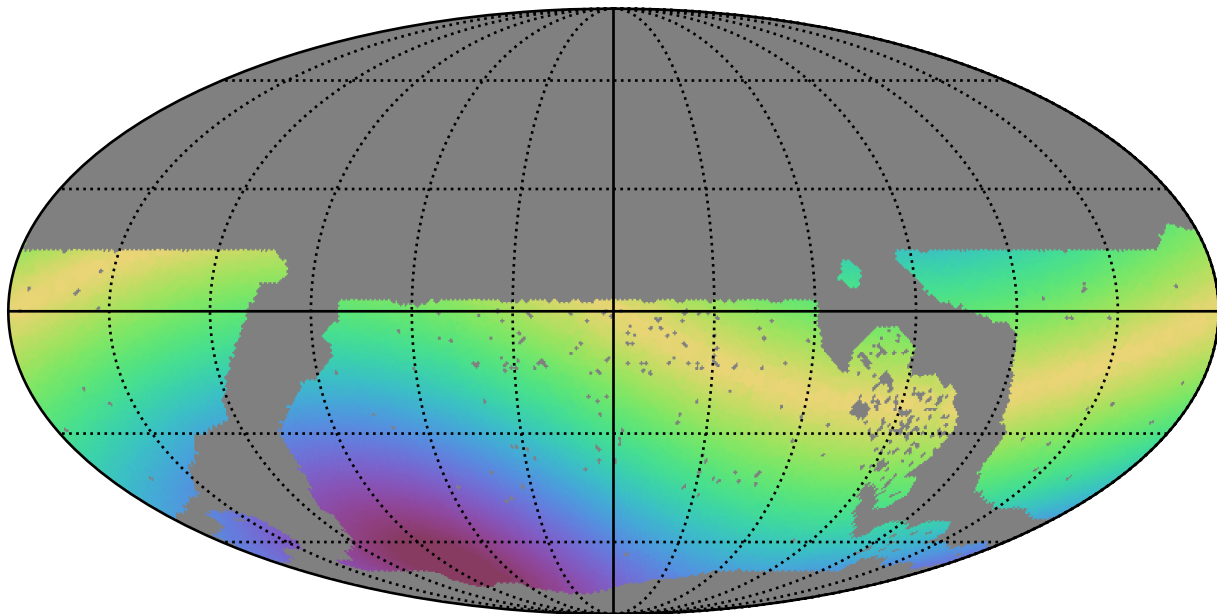
no_long_daily_v3.4_10yrs WFD r band: Max solarElong
