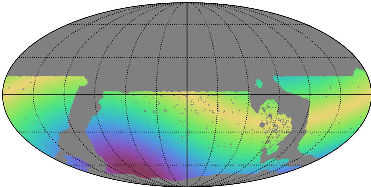
no_long_daily_v3.4_10yrs WFD i band: Max solarElong
