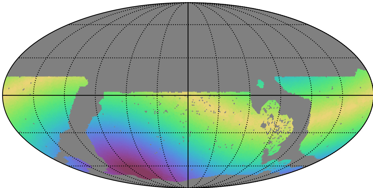
no_long_daily_v3.4_10yrs WFD g band: Max solarElong
