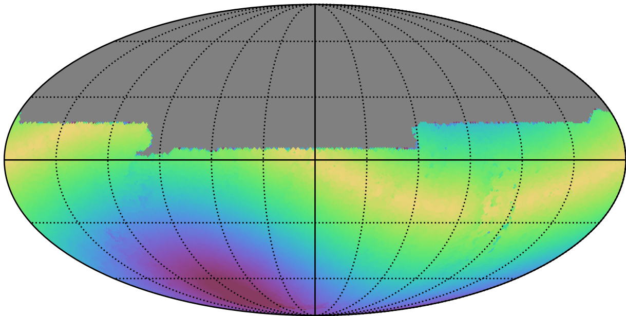
no_long_daily_v3.4_10yrs All sky u band: Max solarElong
