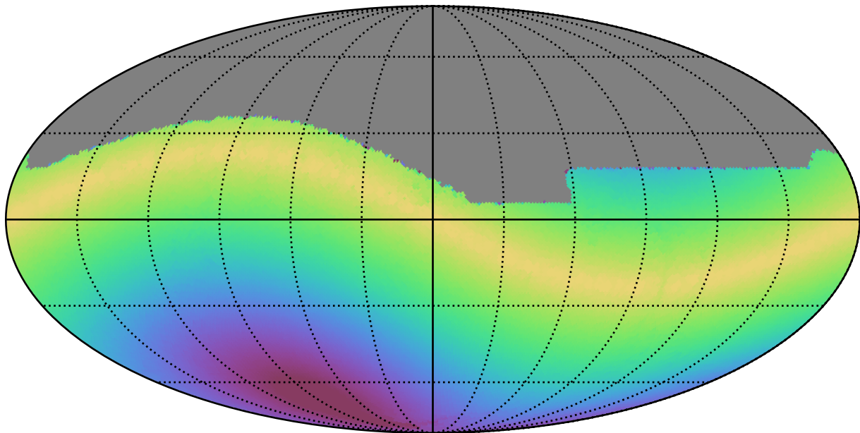
no_long_daily_v3.4_10yrs All sky r band: Max solarElong
