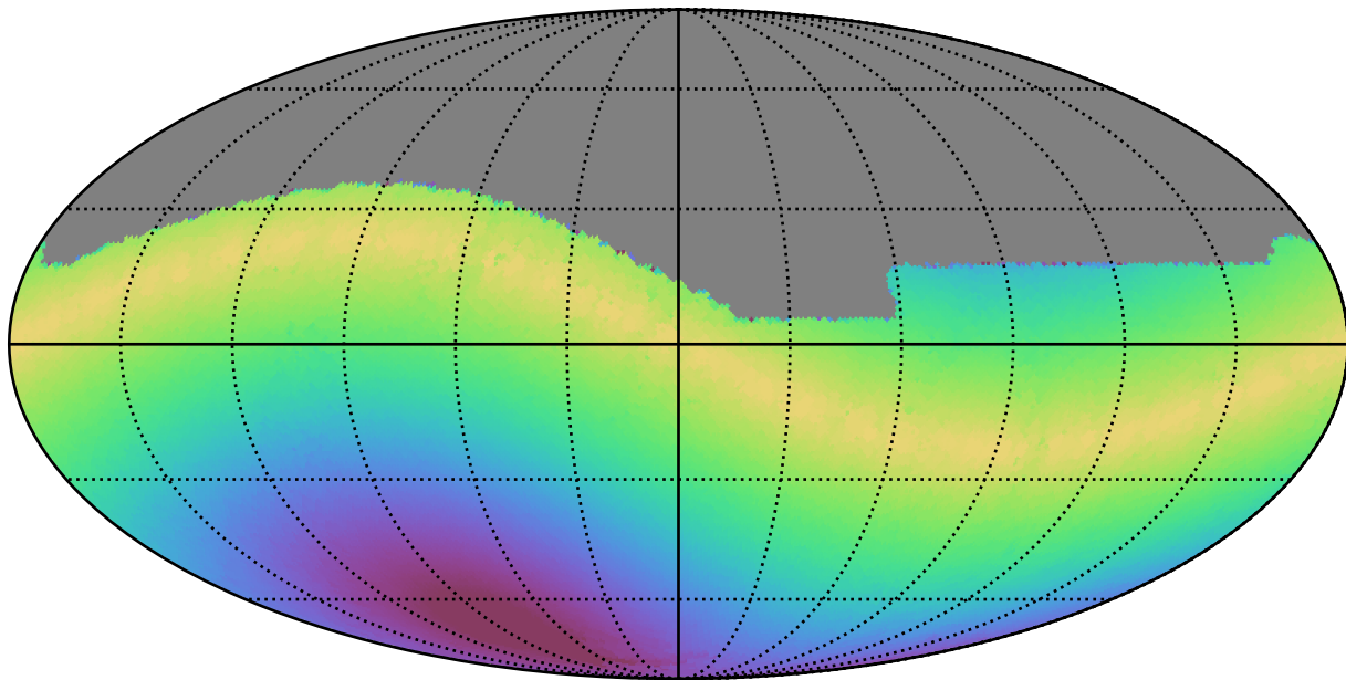
no_long_daily_v3.4_10yrs All sky g band: Max solarElong
