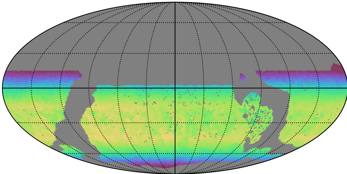
no_long_daily_v3.4_10yrs WFD y band: Max skyBrightness
